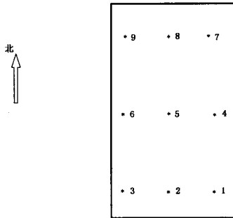
图 B.1 测点布置平面图
