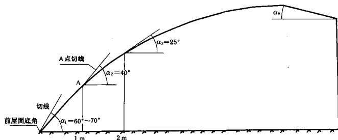
图 1 温室横剖面示意图
