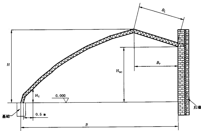
图 C.2 日光温室剖面尺寸示意图
