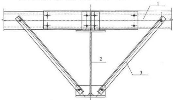
图 7.1.6 屋面斜梁的隅撑 1—檩条; 2—钢梁; 3—隅撑
