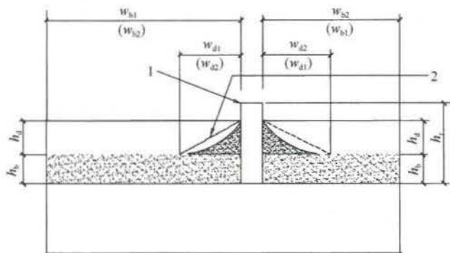
图 4.3.3-4 屋面有突出物雪堆积分布示意
