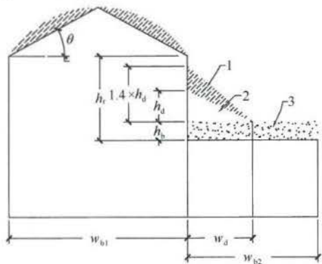
图 4.3.3-3 高屋面雪漂移低屋面雪堆积分布示意
