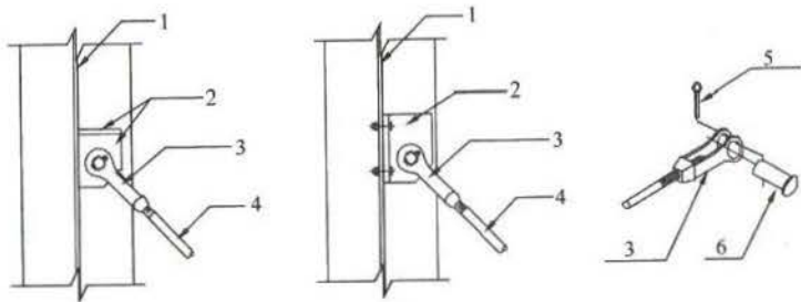
图 8.5.1 圆钢支撑与连接板连接 1—腹板；2—连接板；3—U形连接夹； 4—圆钢；5—开口销；6—插销
