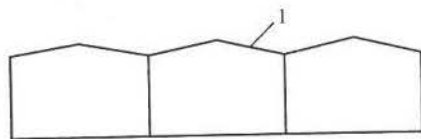
图 4.2.2-5 多跨双坡屋面风荷载系数分区 1—每个双坡屋面分区按图 4.2.2-4c 执行
