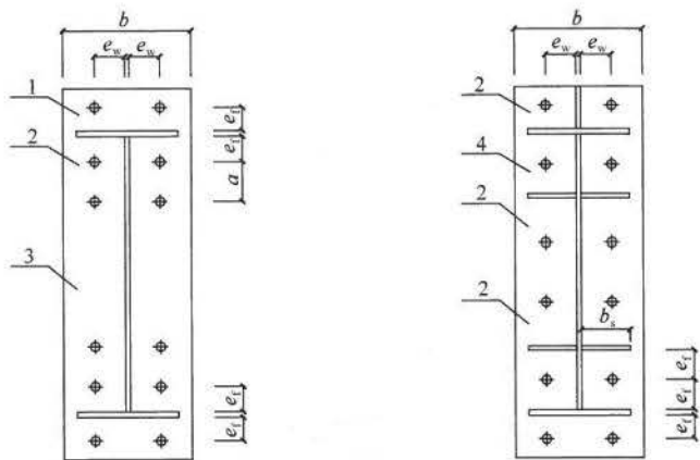
图 10.2.7-1 端板支承条件
