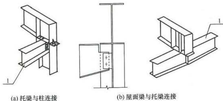
图 10.2.12 托梁连接节点 1—托梁
