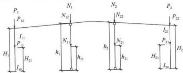
图 A.0.6 带有摇摆柱的框架
