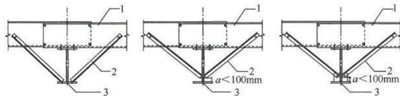
(a) 隅撑与梁柱内翼缘连接 (b) 隅撑与梁柱腹板连接 (c) 隅撑与连接板连接
