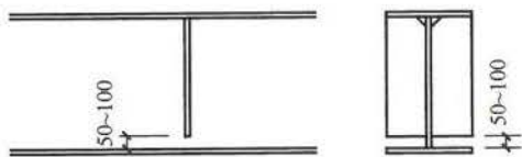
图 10.2.9-2 横向加劲肋设置
