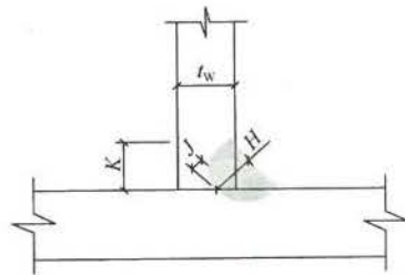
图 10.1.2 单面角焊缝
