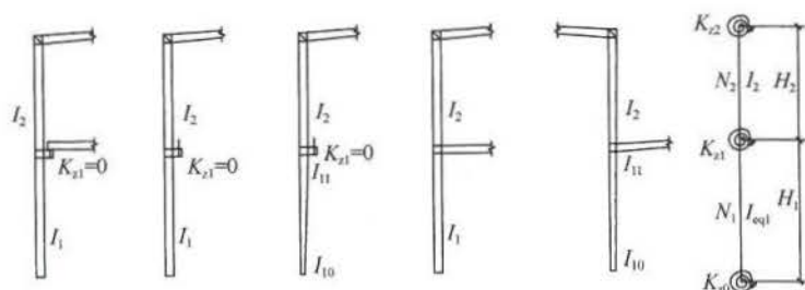
图 A.0.4 变截面阶形刚架柱的计算模型
