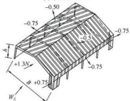
(c) 敞开式房屋纵向
