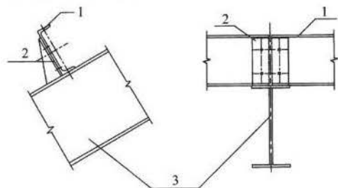
图 9.1.10-1 檩条与刚架斜梁连接
