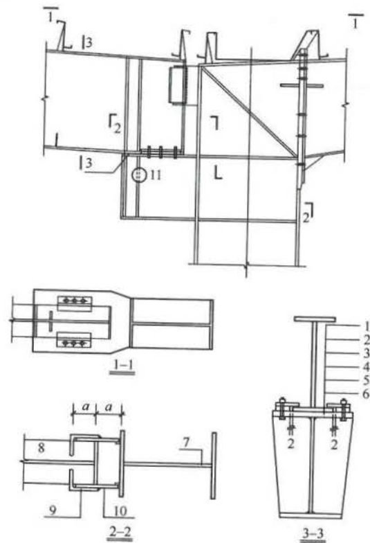
图1 刚架横向温度缝节点图
