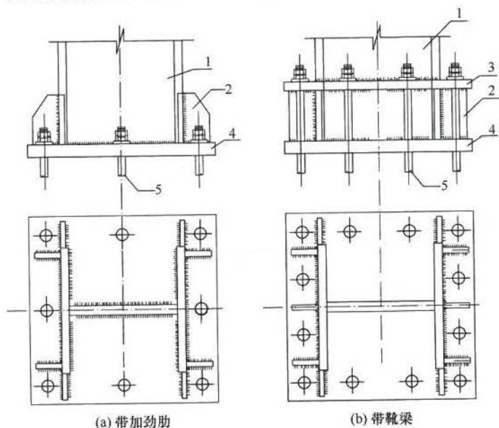
图 10.2.15-2 刚接柱脚
