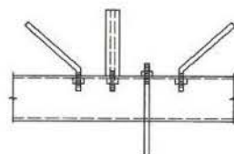
图 9.1.10-3 拉条和撑杆与檩条连接
