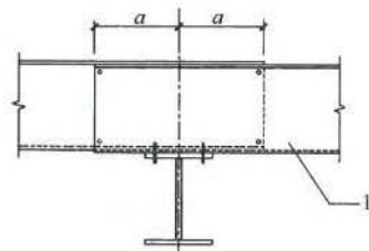
图 9.1.10-2 连续檩条的搭接
