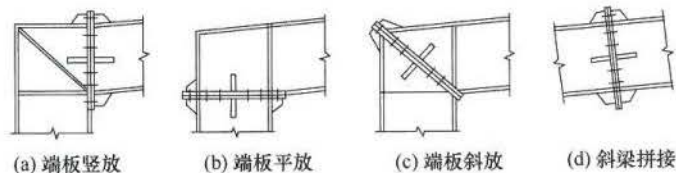
图 10.2.3 刚架连接节点
