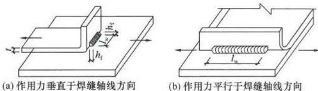
图 10.1.6-1 单边喇叭形焊缝
