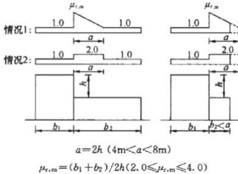
图4 荷载规范中高低屋面雪荷载分布系数规定
