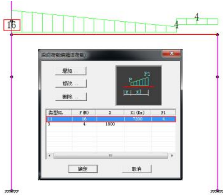
图5 不均匀分布1下程序确定的低跨部位雪荷载
